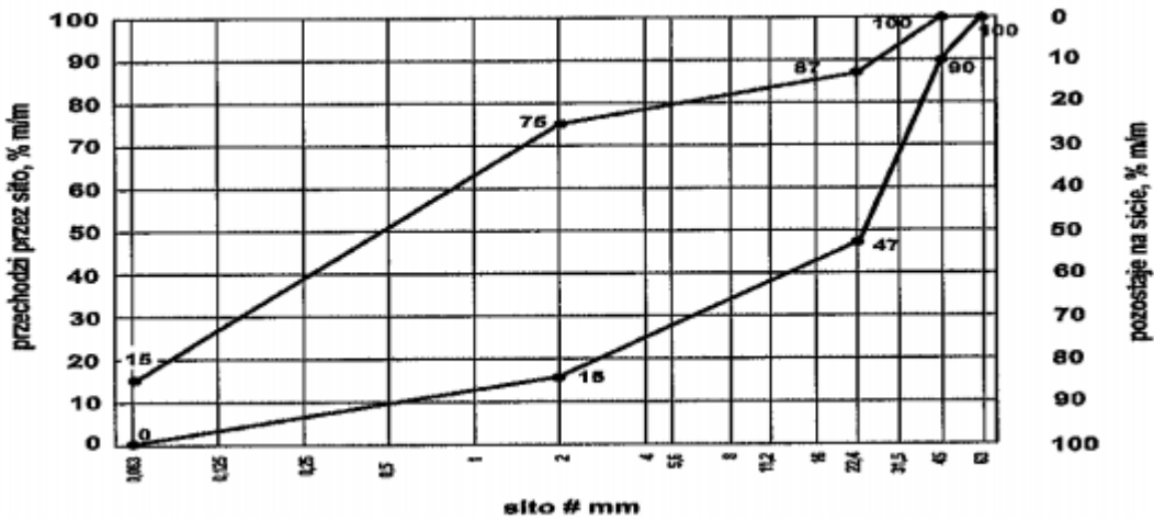
Uziarnienie mieszanki niezwiązanej 0/45 dla górnej warstwy podłoża ulepszonego
