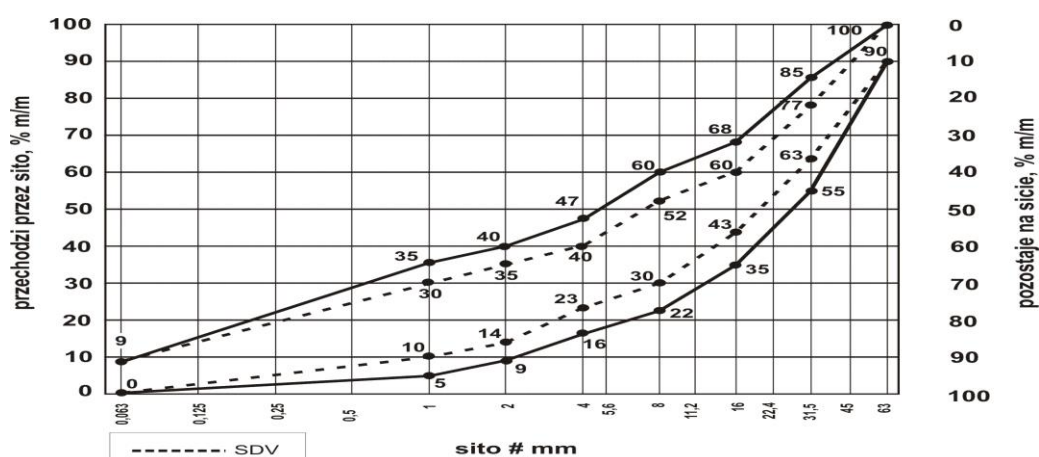
Uziarnienie mieszanki niezwiązanej 0/63 dla podbudowy
