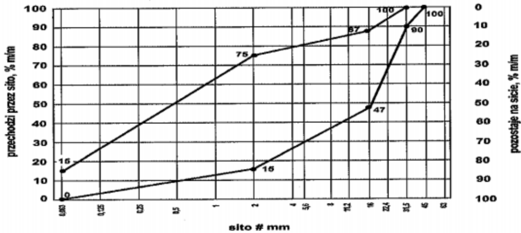
Uziarnienie mieszanki niezwiązanej 0/31,5 dla górnej warstwy podłoża ulepszonego
