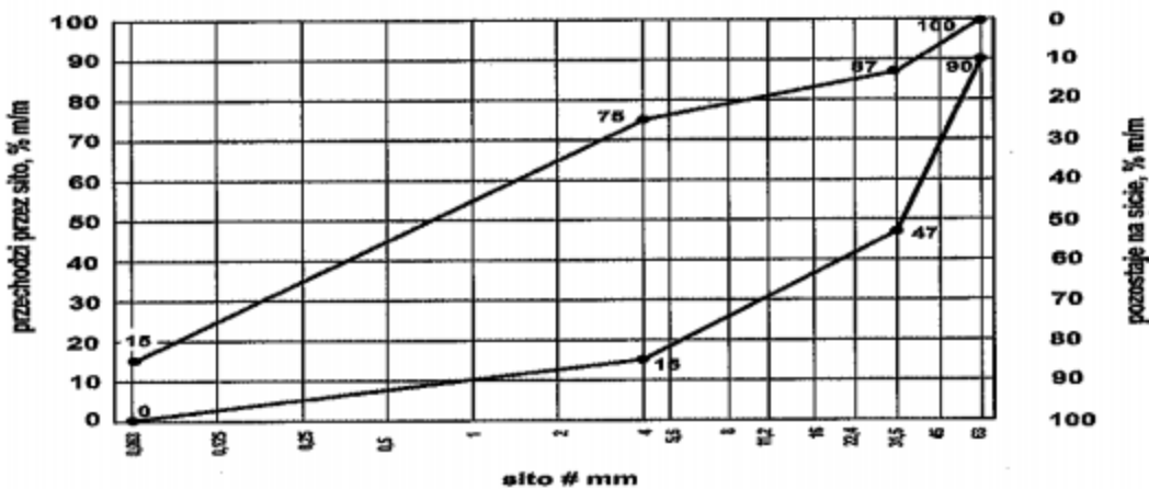
Uziarnienie mieszanki niezwiązanej 0/63 dla górnej warstwy podłoża ulepszonego
