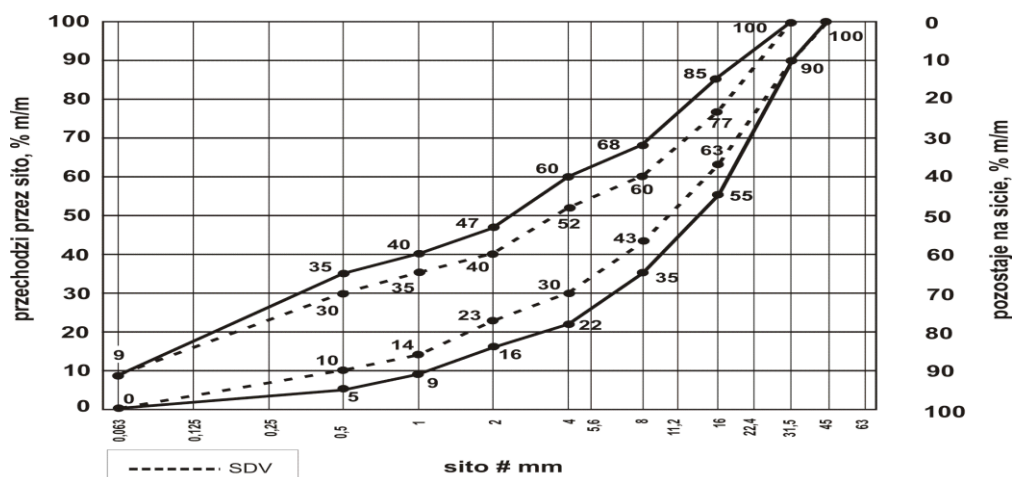
Uziarnienie mieszanki niezwiązanej 0/31,5 dla podbudowy
